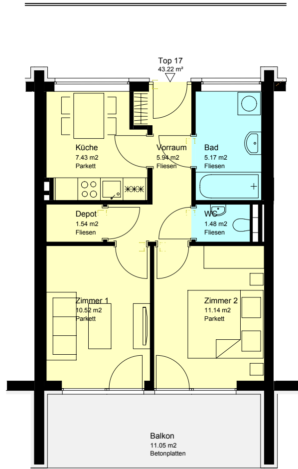
Grundriss
