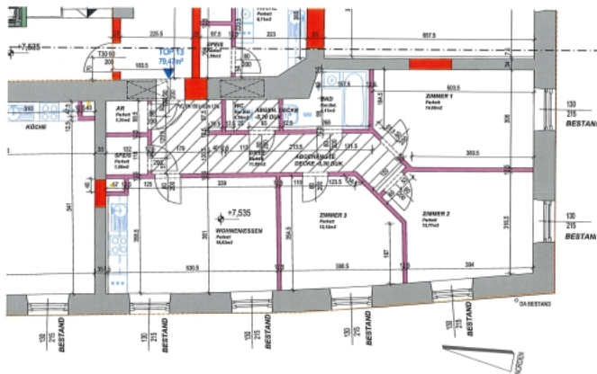
Grundriss M 1:100
