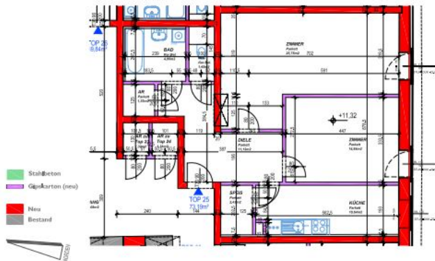
Grundriss M 1:100
